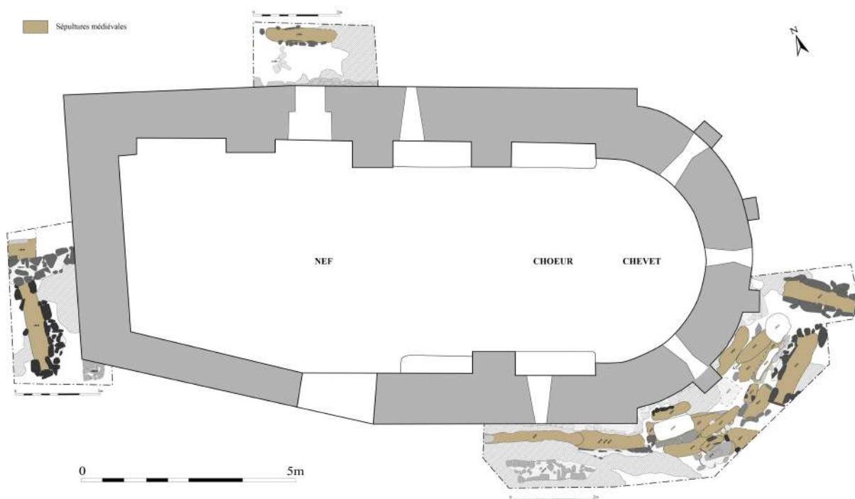
Fig. 2 : Plan de l'édifice et localisation des sondages
